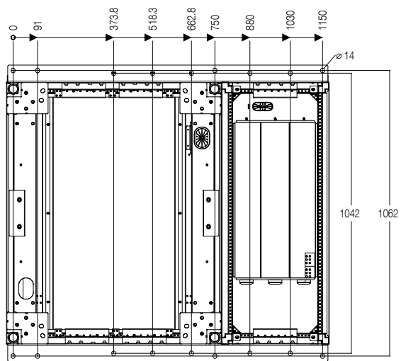
300 - 600 kVA bottom entry
