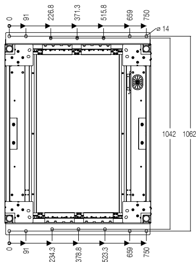
300 - 800 kVA top entry
