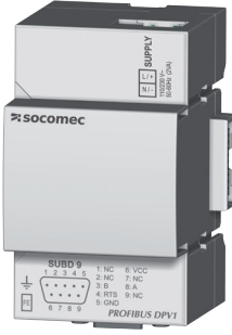
DIRIS O-p PROFIBUS DPV1 Ref. 4829 0034
